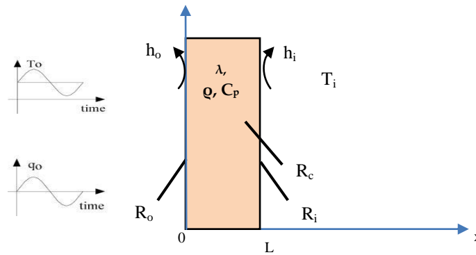
FIGURE 1. Schéma de principe de la géométrie du problème
