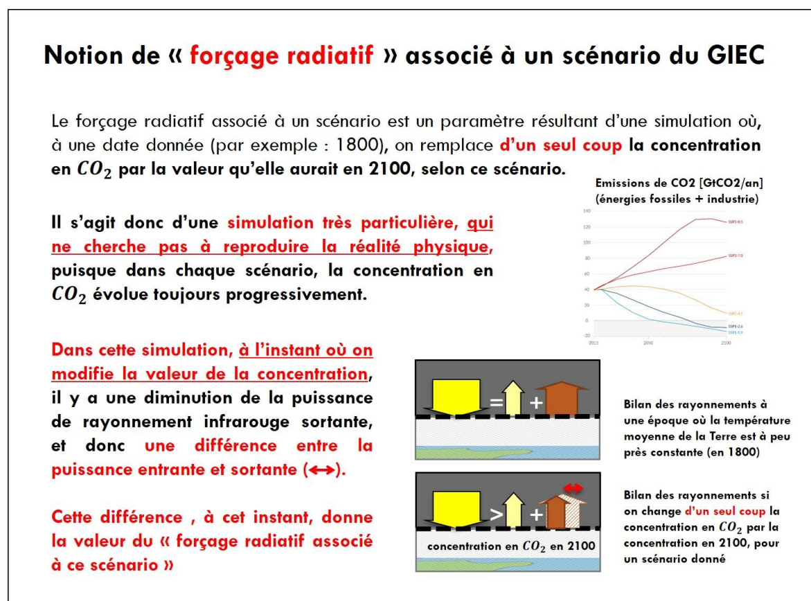
Figure n°20 : Clarification de la définition du forçage radiatif associé au scénarios du GIEC
