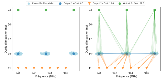
Fig. 11. Résultats de la classification pour l'ensemble d'impulsion 3.
