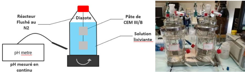
FIGURE 1. Représentation schématique du test de lixiviation réalisé sur échantillons monolithiques
