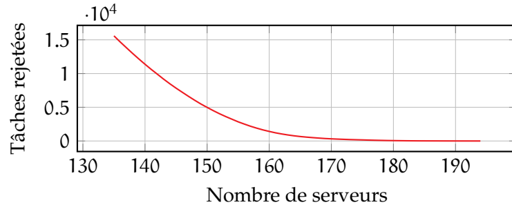
FIGURE 3 – Évolution du nombre de tâches rejetées, en fonction du nombre de serveurs supprimés. m varie de m_{OPT} à m_{min} .
