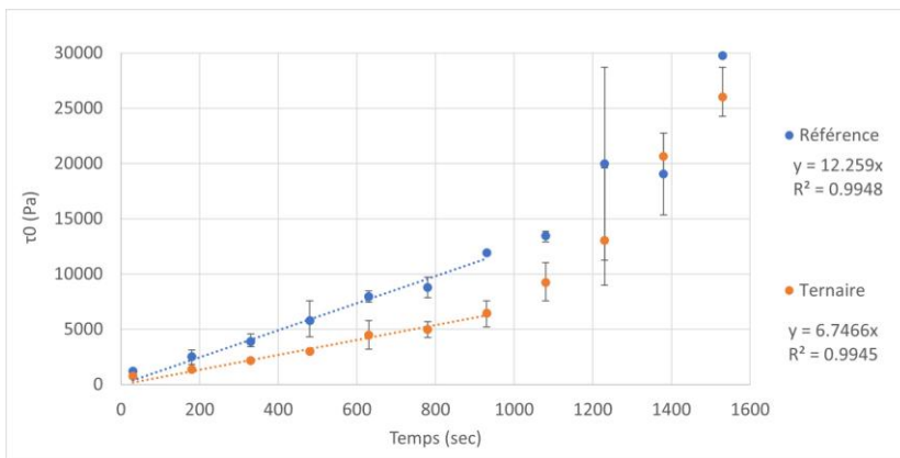
Figure 4. Comparaison des courbes obtenues au fall cône pour le mortier de référence et ternaire
