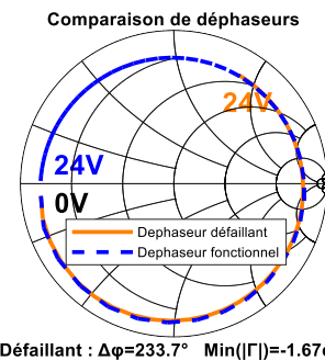
Figure 11 : Mise en évidence d'un déphaseur défaillant
