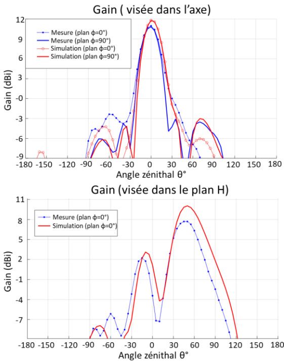
Figure 10 : Gain de l'antenne pour deux visées : [\theta_0=0^\circ] et [\theta_0=50^\circ, \varphi_0=0^\circ]
