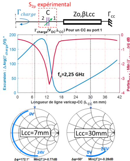
Figure 3: influence de la longueur de ligne Lcc sur le coefficient de réflexion de la varicap en réflexion
