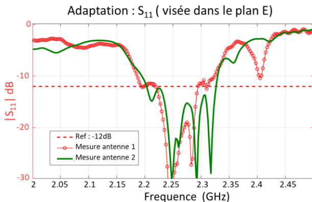
Figure 11 : Comparaison de l'adaptation des deux antennes : visée [\theta_0=40^\circ, \varphi_0=90^\circ]
