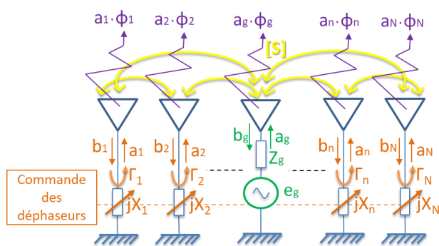
Figure 1 : Architecture d'antenne à éléments parasites pilotés (AEPP)
