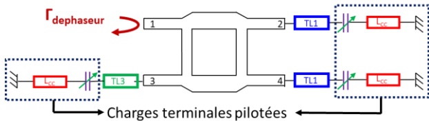
Figure 2 : Schéma de principe du déphaseur en réflexion
