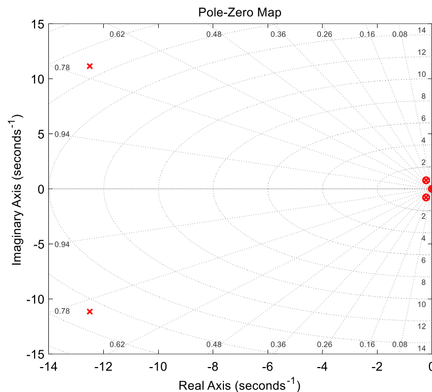
Figure 13. Pole-zero map (x, pole; o, zero).
