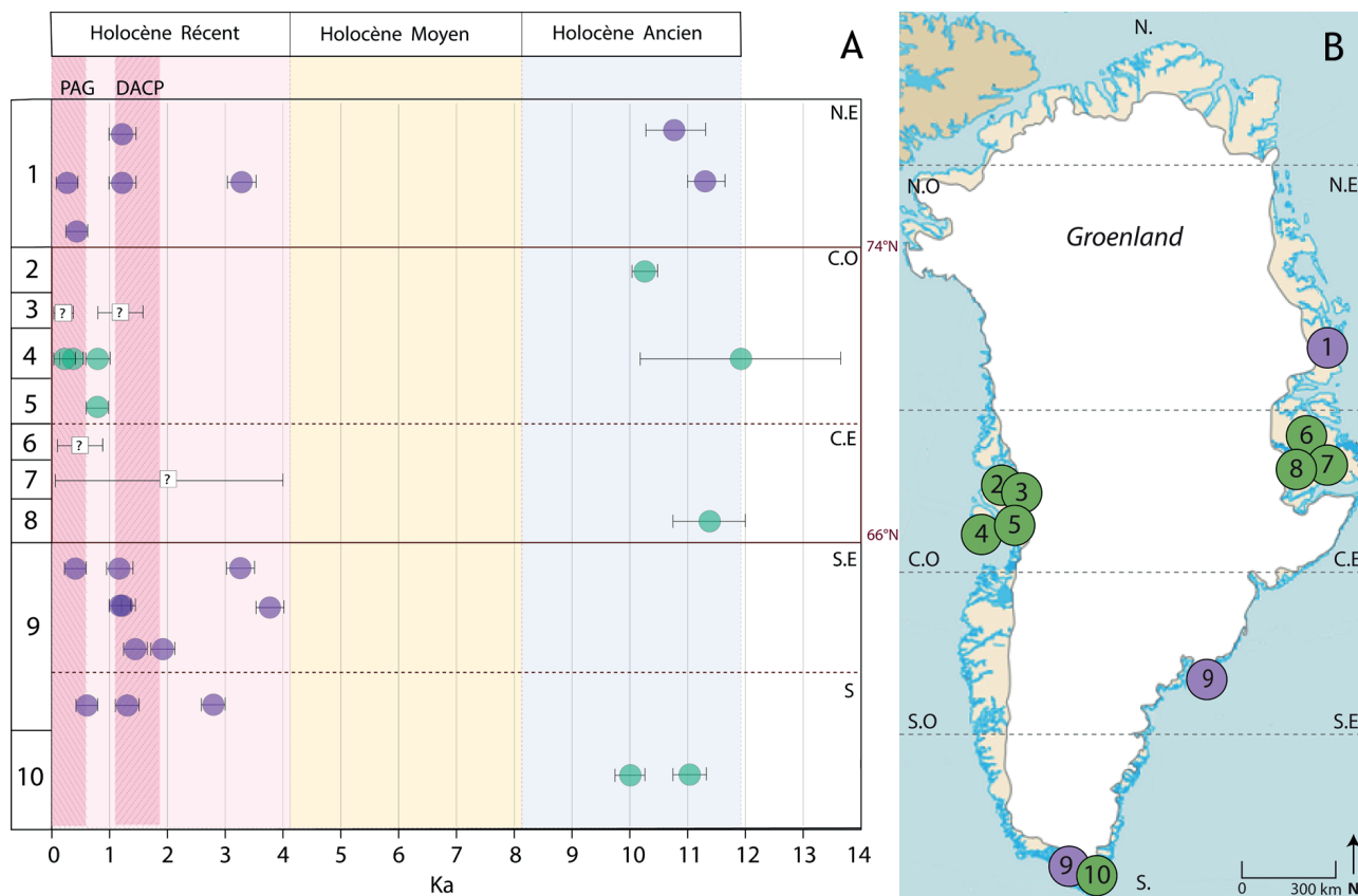
Fig. 2: Résumé des reconstitutions holocènes des glaciers déconnectés de l'inlandsis fondées sur la datation de moraines au Groenland. Les chronologies glaciaires sont présentées du nord au sud (A) et les positions des glaciers représentés sur la carte (B).
