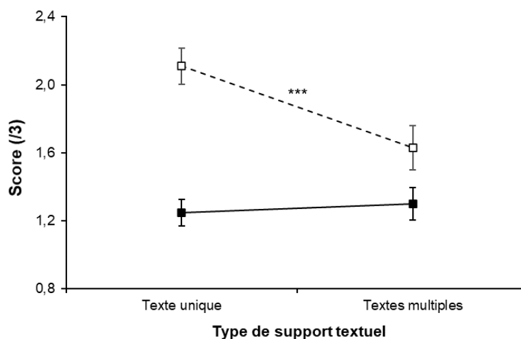
Figure 2. Effet du type de supports textuels sur les questions de bas niveau (□) et de haut niveau (■). (***) p-value au test post hoc de Bonferroni <.001).
