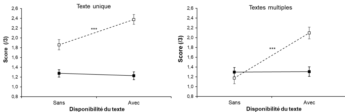
Figure 3. Effet de la disponibilité du texte sur les performances en fonction du type de supports textuels et du type de questions (■ : questions de haut niveau, □ : questions de bas niveau). Les barres d'erreur représentent l'erreur standard. (***) p-value au test post hoc de Bonferroni <.001 ).
