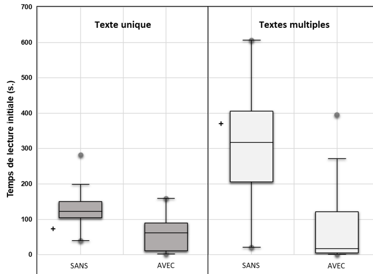
Figure 1 : Diagramme en boîte pour le « temps de lecture initiale » fonction de la disponibilité (avec/sans) et du type de supports textuels. La croix (+) correspond au temps de lecture attendu pour une lecture intégrale avec une fluence de 130 mots/min. Les ronds (●) désignent les valeurs extrêmes.
