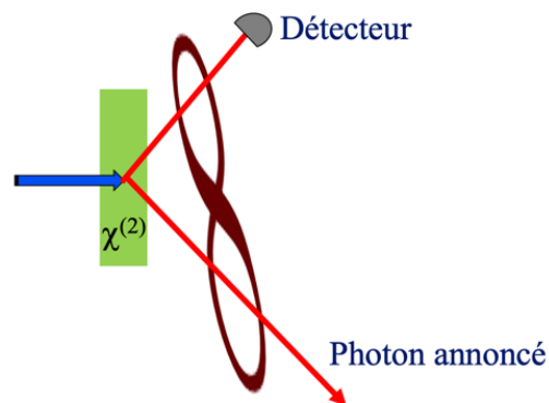
Figure 7 : Schéma de principe de la création d'un photon annoncé (mêmes conventions que pour la Fig. 6).
