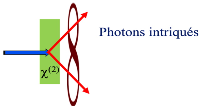
Figure 6 : Schéma de principe de la création de photons intriqués par interaction paramétrique : un faisceau laser (à gauche, en bleu) est décomposé dans un milieu non linéaire (en vert) en deux faisceaux de fréquence moitié (en rouge, à droite). La double boucle curviligne symbolise l'intrication entre les deux composantes.
