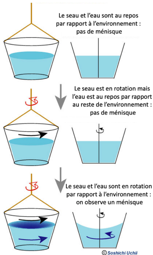
Figure 1 : Expérience de pensée dite du « seau de Newton » :
