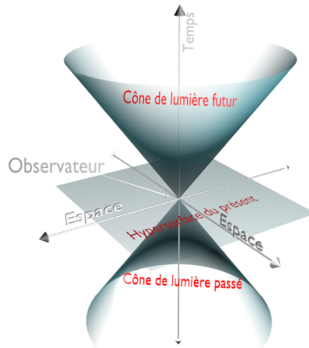
Figure 2 : Cône de lumière dans l'espace-temps de la relativité restreinte. L'extérieur du double cône constitue l' ailleurs absolu , inaccessible à toute action à distance (Origine : Wikimedia)
