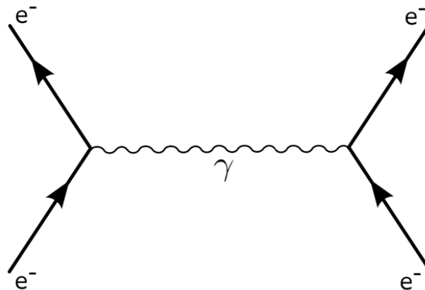
Figure 4 : Diagramme de Feynman élémentaire : représentation de l'action à distance entre deux électrons supposément isolés par échange d'un photon virtuel \gamma (source : Wikimedia)
