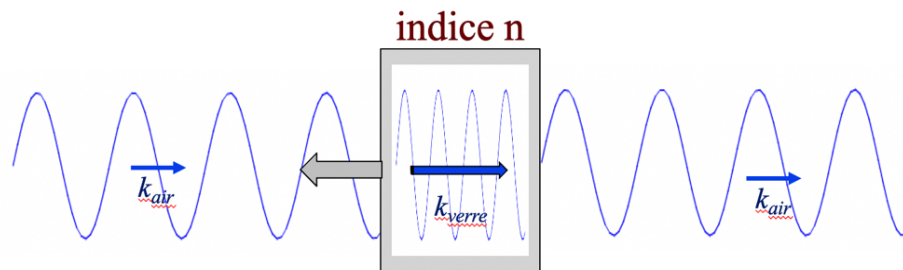
Figure 5 : Lorsqu'un photon de fréquence \nu traverse un diélectrique (e.g. une lame de verre) d'indice n ( \approx 1,5 ), son impulsion canonique ( p_{\text{verre}} = n h \nu / c ) y est plus grande que dans l'air ( p_{\text{air}} = h \nu / c )
