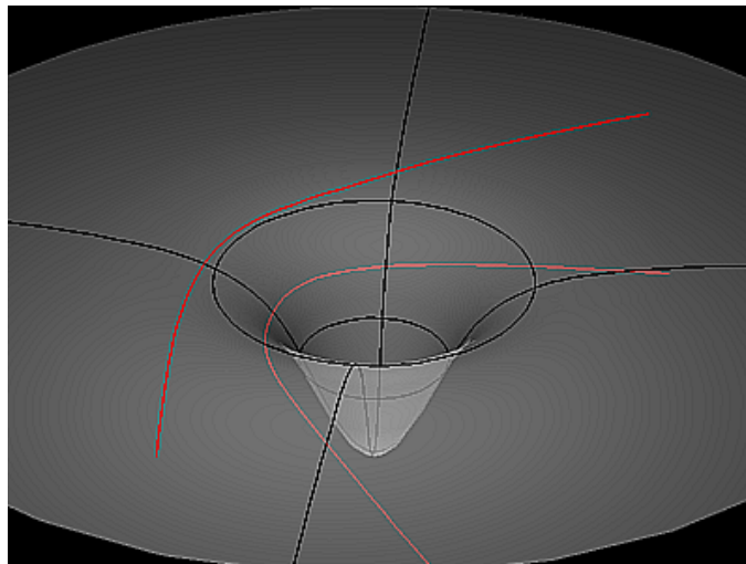
Figure 3 : Géodésiques dans un espace-temps courbe (source : Wikimedia)
