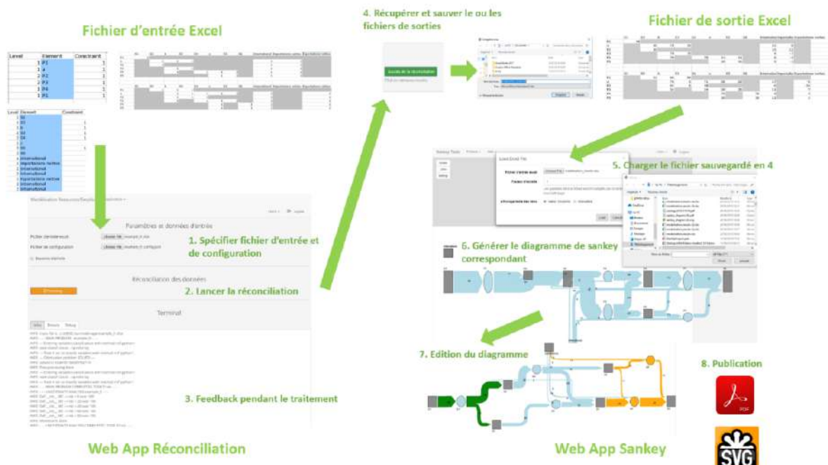
Figure 14 : Présentation des principaux éléments et enchainements des Web App réconciliation et Sankey
