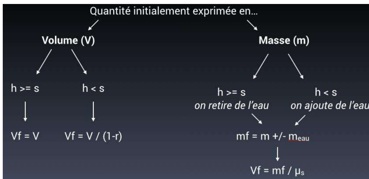
Figure 4: Principe de conversion en m3f. H : taux d'humidité, s : taux de saturation, \mu_s : masse volumique de l'essence de bois au point de saturation, V : volume plein du produit, Vf : volume exprimé en m3f. Subtilités : (i) si le volume du produit considéré est un volume apparent, il faut d'abord le convertir en volume de bois plein, (ii) si le produit contient d'autres substances que du bois (par exemple de la colle), il faut tout d'abord soustraire la masse correspondante.
