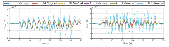
(a) CoM x error. (b) CoM y error.
