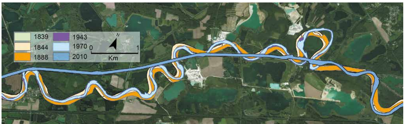
Figure 37. Évolution du tracé en plan entre 1839 et 2010, issue de l'analyse des cartes anciennes (fonds de carte © IGN).
