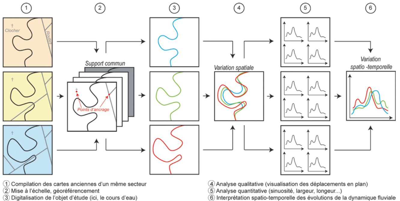
Figure 36. Démarche méthodologique pour le traitement et l'analyse des cartes anciennes. Schéma simplifié, adapté de la chaîne de traitement développée par Miramont et al. (1998).
