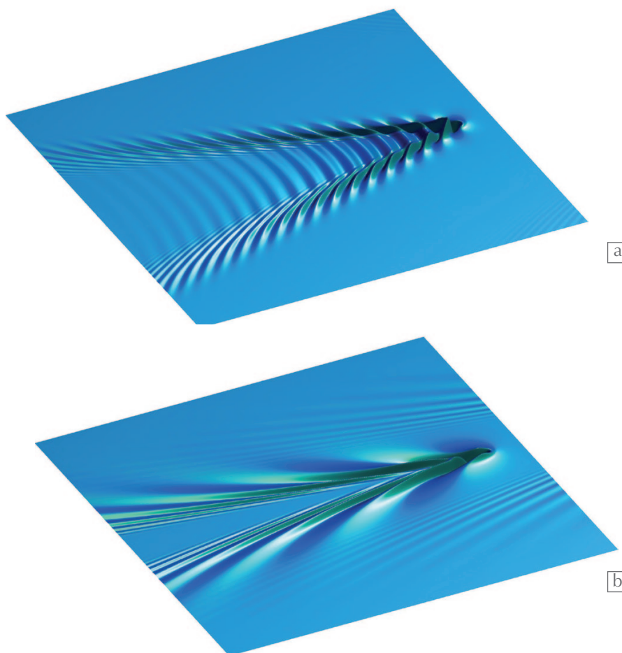
5. Simulation numérique d'un sillage induit par une perturbation de pression gaussienne se déplaçant à nombre de Froude \text{Fr} = 0,5 (a) et 1,5 (b).
