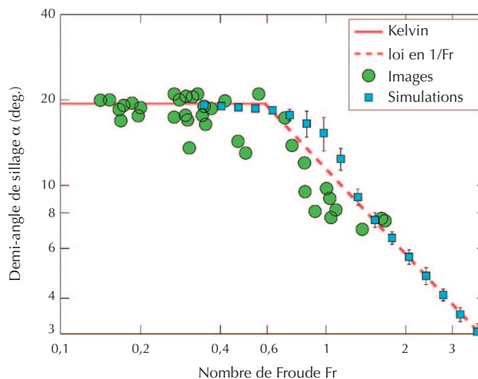
4. Évolution du demi-angle \alpha du sillage observé en fonction du nombre de Froude \text{Fr} = U/(gL)^{1/2} , montrant une transition entre le régime de Kelvin (angle constant égal à 19,47^\circ ) et le régime en 1/\text{Fr} à haute vitesse.
