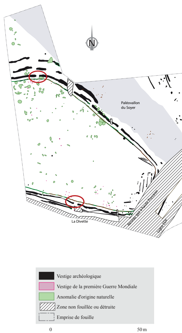
FIG. 7. Plan des structures de l'enceinte de Passel « Le Vivier » (Oise).
