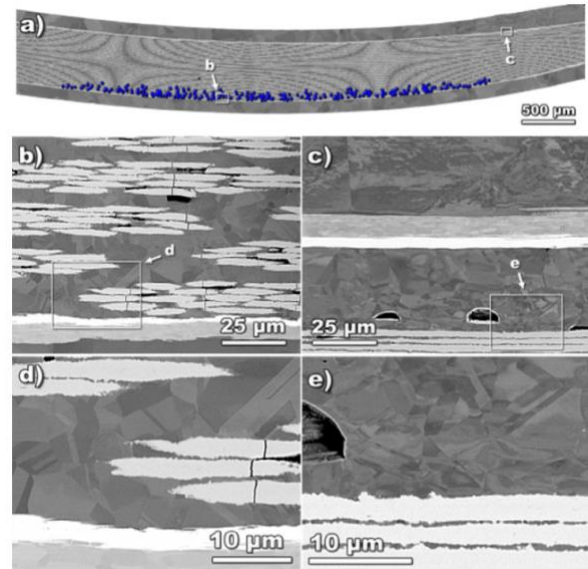
Figure 15 : Coupe longitudinale d'un brin Nb_3Sn - IT extrait d'un test de chargement cyclique électromagnétique de conducteur CICC pour ITER dans le cadre d'une campagne de test des dégradations cycliques [20]
