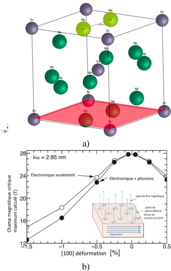
Figure 6 : a) Cristallographie du composé intermétallique Nb 3 Sn (maille cubique composée de 2 atomes d'étain et de 6 atomes de niobium dénotée cP8 ou A15). b) Champ magnétique critique maximum en fonction de l'état de déformation dans Nb 3 Sn (adapté de [7]).
