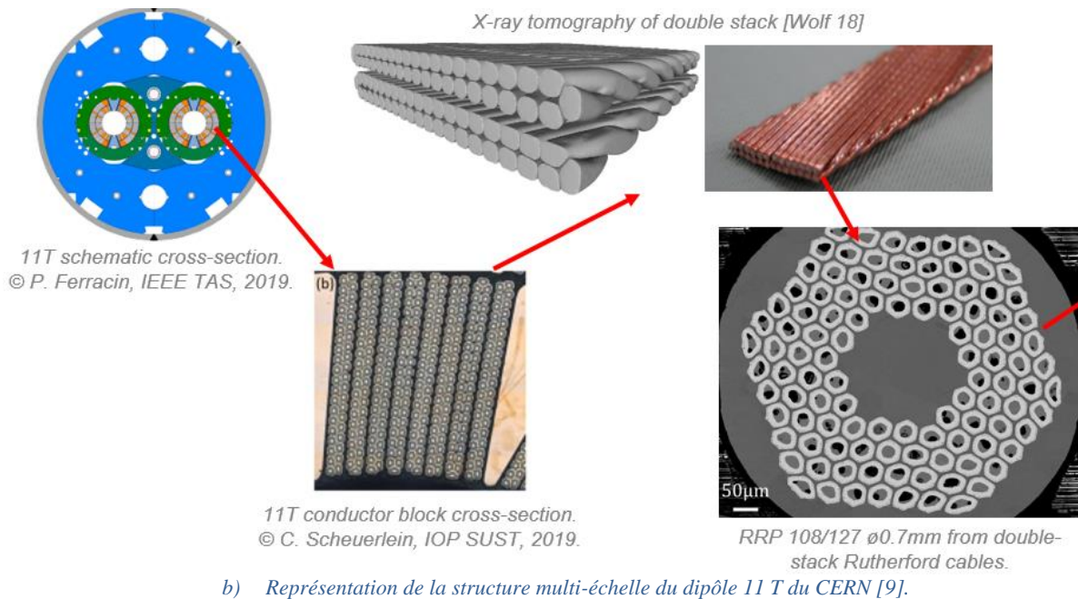
Figure 7 : Représentation de la complexité et de la structure multi-échelle de l'utilisation des conducteurs supraconducteurs dans le cadre du projet ITER et des aimants d'accélérateurs
