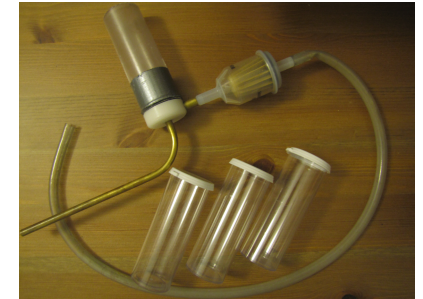
Figure 6 : Aspirateur à insectes
