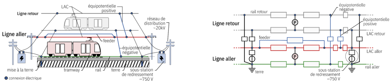
Figure 1 : a. Infrastructure électrique d'une ligne de tramway – b. Modèle de circuit électrique équivalent
