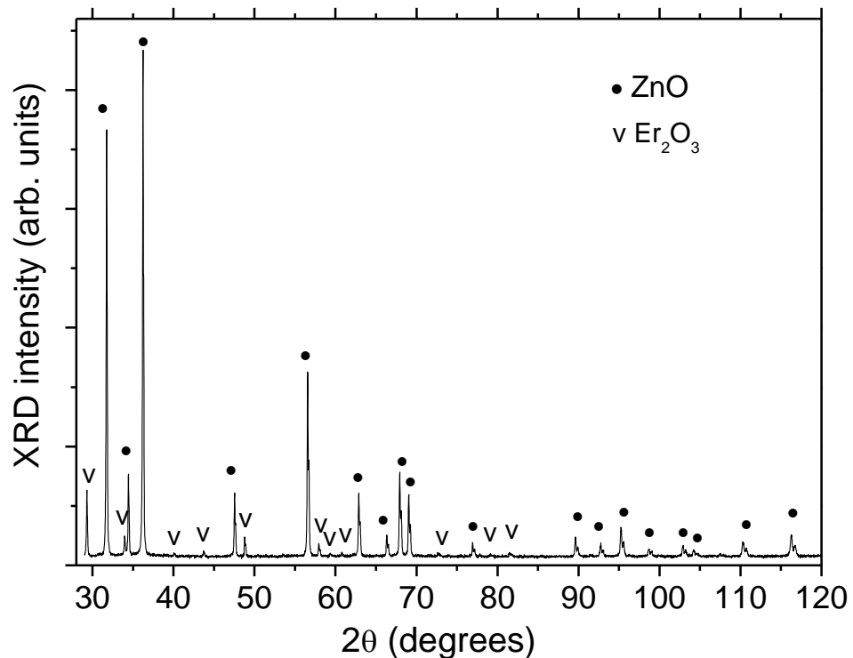
Fig. 1513. XRD pattern of ZnO:5% Er optical ceramic.
