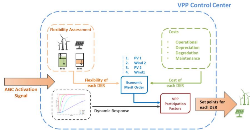
Fig. 3: VPP-CS scheme
