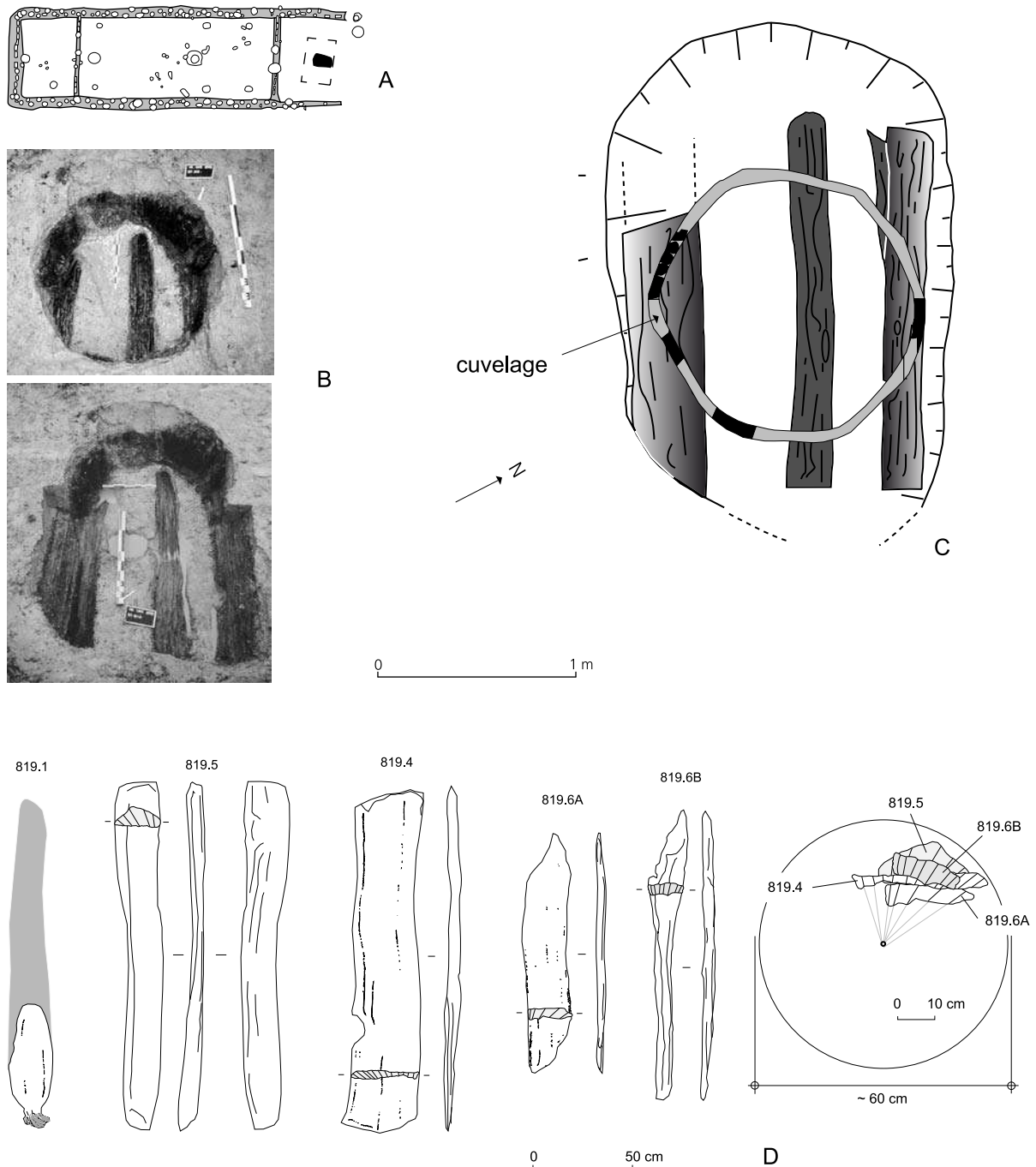
Fig. 4. A : Localisation. B : Photographies. C : Relevés de la structure 819. D : Principaux éléments en bois issus de la structure 819 et remontage dendroarchéologique (V. Bernard).
