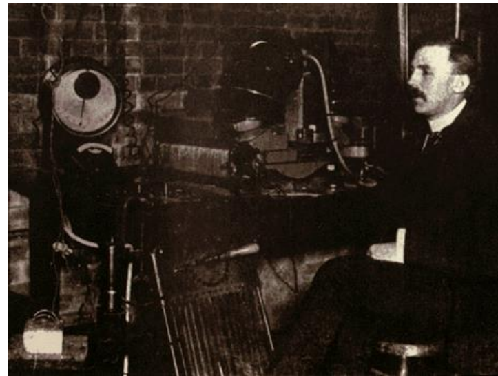
1911, Ernest Rutherford met en évidence le noyau atomique constitué de protons
