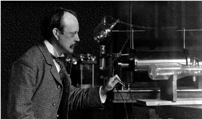
1896, Joseph John Thomson découvre l'électron
