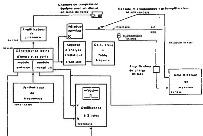
Figure 4 Chaîne d'émission-réception.
