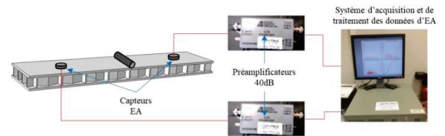
Figure 4 – Dispositif d'émission acoustique.
