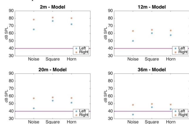
Figure 8 – Niveaux de diffusion des sources statiques et du bruit de fond (extérieur) déjà utilisé dans l'expérience A.
