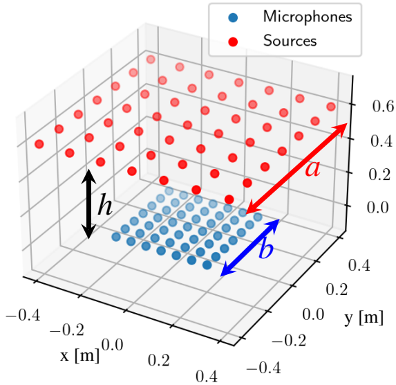
FIGURE 1 – Exemple de configuration de système : 49 sources, a = 80 cm et 81 microphones, b = 40 cm, h = 60 cm
