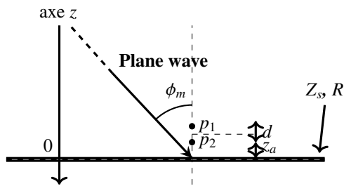
FIGURE 2 – Schéma du doublet microphonique avec une source placée au-dessus d'un plan d'impédance Z_s .
