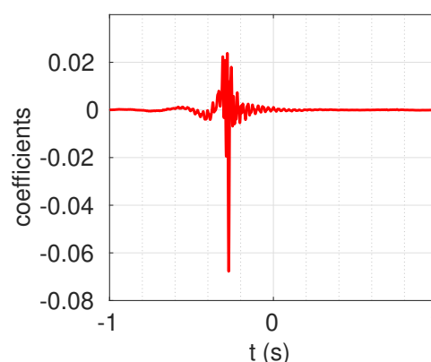
FIGURE 7 – RI d'un filtre égalisateur de phase dans la bande (3-80 Hz), avec compensation de la phase du filtre passe-bande
