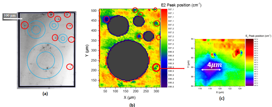
Figure 1 : (a) Image par Cathodo-luminescence montrant des amas de dislocations (entourés en rouge) réalisée avant le dépôt des contacts Schottky. (b) Cartographie micro-Raman de la position du pic E_2^h montrant la présence des mêmes amas de dislocations. Les cercles noirs correspondent aux métallisations des contacts Schottky de diamètres respectifs 200 \mu\text{m} , 100 \mu\text{m} and 50 \mu\text{m} . (c) Zoom sur un amas de dislocations.
