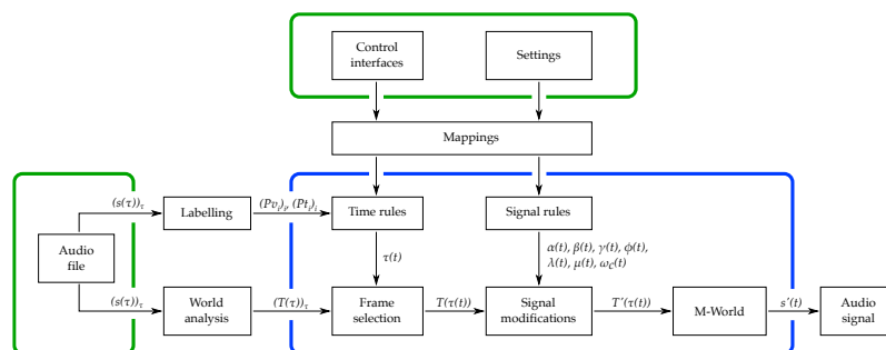
Figure 2 : Schéma de principe de Voks. En haut le contrôle gestuel et l'interface utilisateur ; au centre le synthétiseur par échantillonnage ; à gauche la base de données d'échantillons étiquetés (Locqueville et al. 2020)
