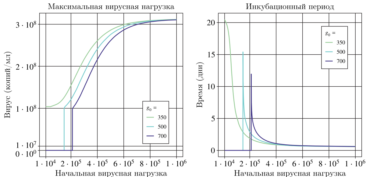
Рис. 6. Максимальная вирусная нагрузка (слева) и инкубационный период (справа) как функции начальной вирусной нагрузки при численном моделировании системы (1)–(6). Вертикальные линии — это значения вирусной нагрузки, при которых сходимость решения меняется с первой стационарной точки на третью. Фиолетовая линия соответствует моностабильному случаю с одной стационарной точкой с большим значением вирусной нагрузки
