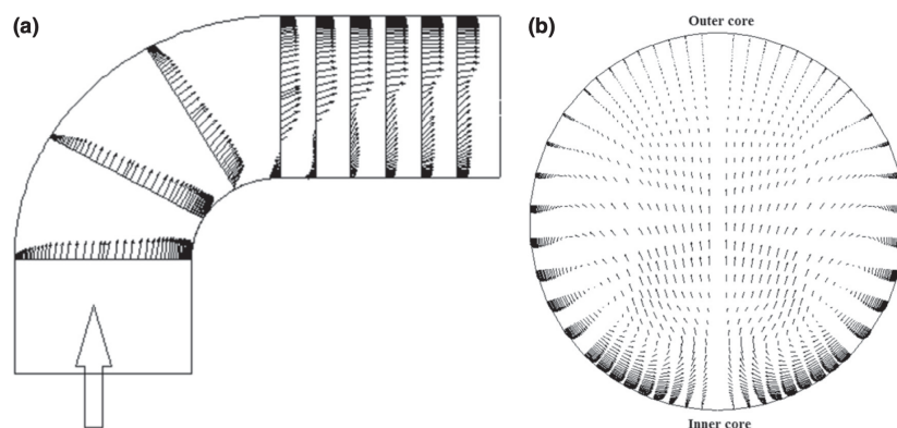
FIGURE 1 – Écoulement à travers un coude 90° : vecteurs vitesses normalisés. (a) plan de symétrie (b) section à 90°. Extrait de de Dutta et al. [10]
