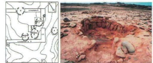
Antiguas aldeas de pescadores de entre 6500 y 4000 años de antigüedad: (izquierda) croquis del sitio de Chacaya 2; (derecha) fotografía del sitio de Aguada de Gualaguala 04.
