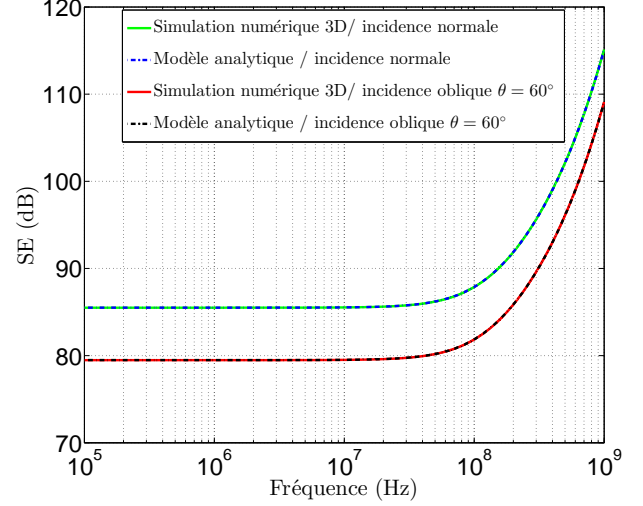
FIGURE 2. Comparaison de SE d'un plan métallique par simulation numérique 3D et le calcul analytique.
