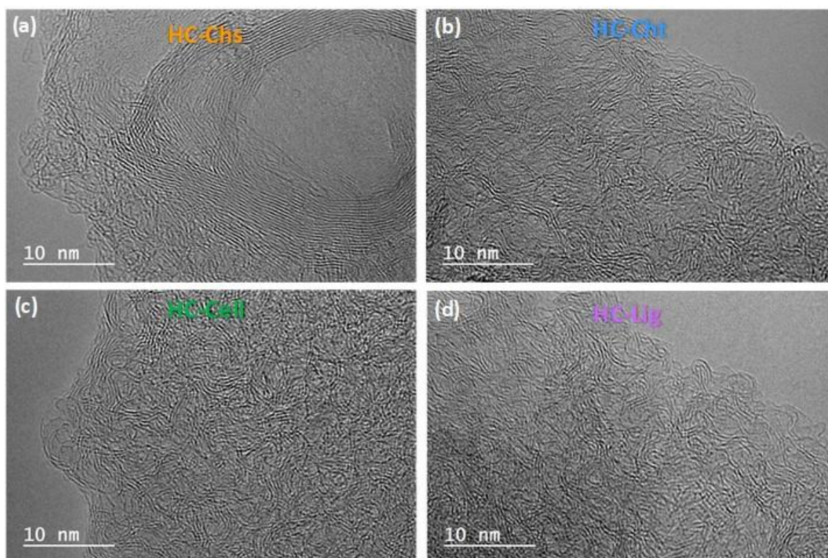
Figure 2: HRTEM images of hard carbon materials: (a) HC-Chs, (b) HC-Cht, (c) HC-Cell and (d) HC-Lig.
