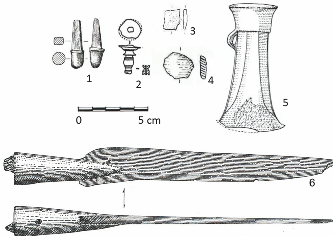
Fig. 10. Objets en fer des dépôts du Bronze final atlantique 3 (1 et 2, objets bimétalliques bronze et fer ; 5, large tache d'oxyde de fer sur une hache à douille en bronze). 1. le Petit Villatte à Neuvy-sur-Barangeon, Cher (d'après Cordier, 1996) ; 2. Haute Queue à Lacroix-Saint-Ouen, Oise (d'après Blanchet, 2001) ; 3. Champ de la Villate à Challans, Vendée (d'après Verney, 1990) ; 4-5. Vénat à Saint-Yrieix, Charente (d'après Coffyn et al. , 1981), 6. les Isles, Chabris, Indre (d'après Cordier, 2009).
