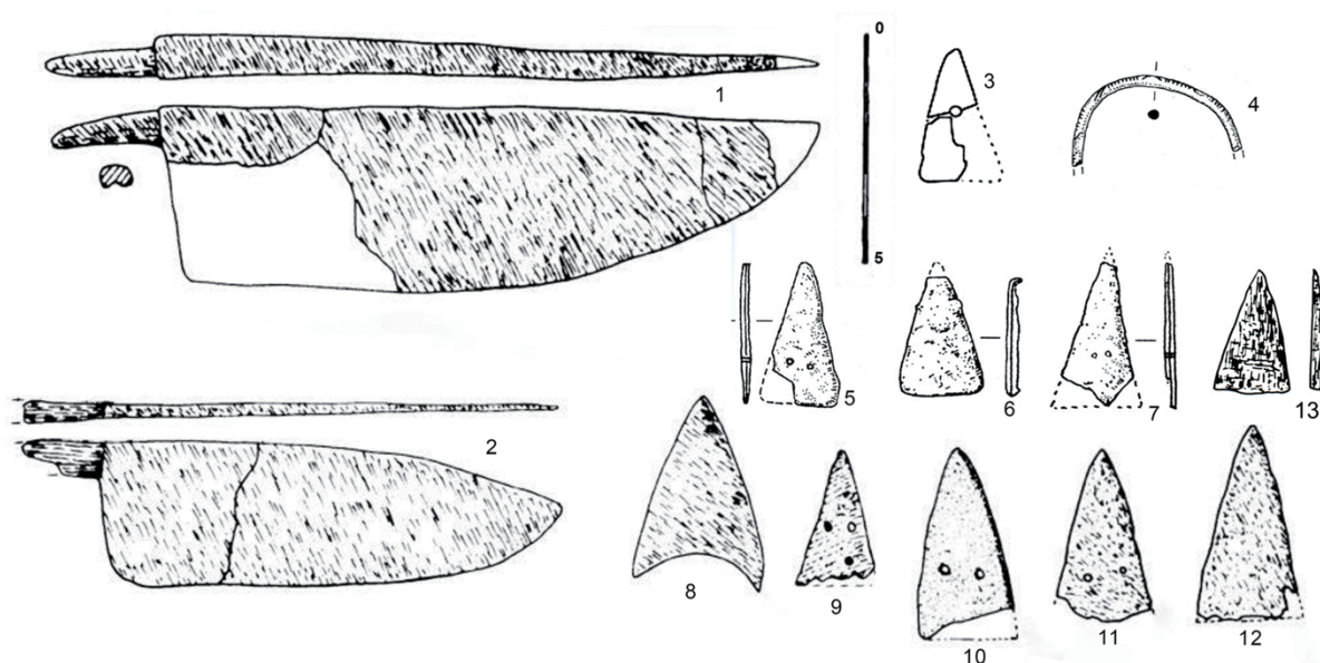
Fig. 8. Objets en fer venant d'habitats et de sépultures. 1, 2, 8-12. grotte du Quéroy, Chazelles, Charente (d'après Gomez de Soto et Kerouanton, 1991) ; 3. Épogny, Couches, Saône-et-Loire (d'après Thévenot, 1985) ; 4. tumulus B de La Chaume, Ivry-en-Montagne, Côte-d'Or (d'après Olivier et Triboulot, 1999) ; 5-7. La Montagne de Myard, Vitteaux, Côte-d'Or (d'après Nicolardot, 2003) ; 13. tumulus du Clos du Biberon, Aslonnes, Vienne (d'après Pautreau, 1984).
