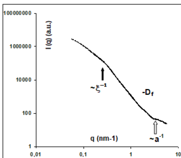
Figure 75: Courbe SAXS typique d'un andosol
