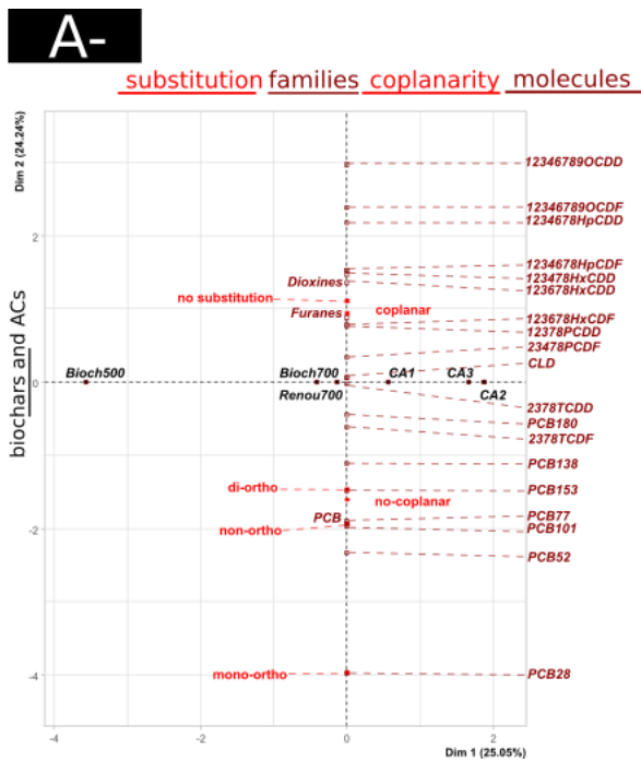
Figure 41: Dispersion des variables A-qualitatives et B-quantitatives décrivant les charbons et biochars (Dim1) et les molécules (Dim2)
