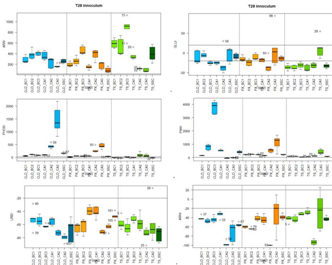
Figure 65: Evolution des activités enzymatiques T28/T0: %évolution par rapport T0 (vert : sols sans contaminant, bleu : sols avec chlordécone, orange : sol avec PCB, couleur plus foncée : modalité sans matrice carbonée)
