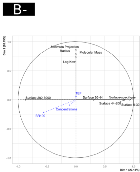
Figure 41: Dispersion des variables A-qualitatives et B-quantitatives décrivant les charbons et biochars (Dim1) et les molécules (Dim2)
