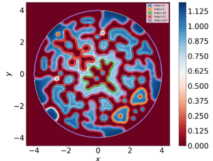
(D) The vortex sheets' indices of the second component.
