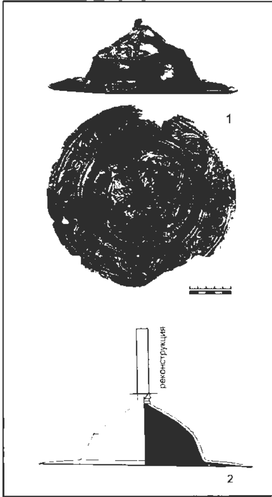
Fig. 4. Umbo de la tombe d'Iulius Kallisthénès (d'après Sharov et Choref 2015, fig. 7).
