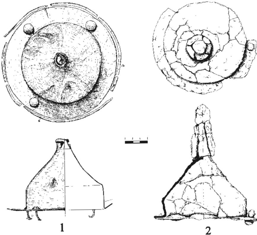
Fig. 7. Umbos de la nécropole de Neizats. 1: tombe 152; 2: tombe 306 (d'après Khrapunov 2011, fig. 25).
