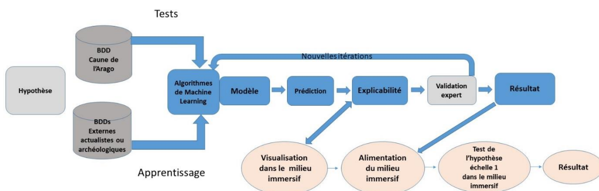
Figure 2 - workflow du test d'hypothèses dans la plateforme SCHOPPER
