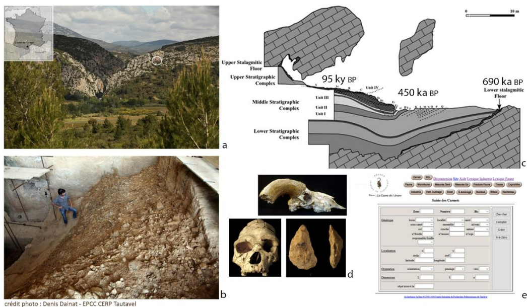
Figure 1 - Le site pléistocène de la Caune de l'Arago à Tautavel. a) Situation et contexte du site. b) Vue d'un sol archéologique. c) Coupe longitudinale de la grotte. d) Découvertes exceptionnelles - crâne de Mouflon, face Arago XXI, biface. e) capture d'écran de l'interface d'interrogation de la base de données actuelle.
