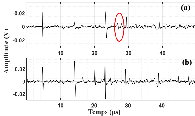
Figure 12 : Signaux acquis lorsque la détection et les sources sont positionnées au niveau 0 (a), au niveau 1 (b).
