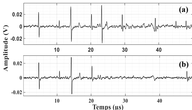
Figure 10 : Signaux détectés avec (a) et sans (b) source S_3 .
