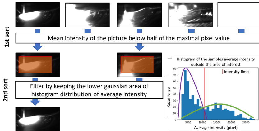
Fig. 3. Numerical sort
