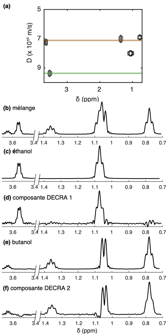
Figure 4 Les données RMN DOSY ultrarapide peuvent être analysée avec une approche univariée, illustrée en (a) dans le cas d'un mélange d'éthanol et de butanol. Dans ce cas, les signaux qui se recouvrent à 1.05 ppm ne sont pas séparés, et le coefficient de diffusion estimé a une valeur intermédiaire entre les valeurs obtenues pour l'éthanol et pour le butanol. Avec un traitement multivarié (l'approche DECRA, on peut séparer les spectres 1D des deux molécules : (b) spectre du mélange ; (c) spectre de l'éthanol seul ; (d) premier spectre issu de l'analyse DECRA de données RMN DOSY ultrarapide ; (e) spectre du butan-1-ol. (f) second spectre issue de l'analyse DECRA.
