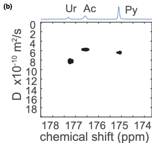
Figure 5 La polarisation dynamique nucléaire (DNP) permet d'accroître l'intensité des signaux RMN d'un facteur pouvant dépasser 10 000. Comme décrit en (a), l'échantillon est placé à très basse température, irradié avec des micro-ondes, puis dissout et transféré vers les spectromètres RMN pour enregistrer des spectres. La combinaison de la RMN diffusionnelle ultrarapide et de la DNP permet d'observer d'autres noyaux tels que le carbone-13, comme illustré en (b) pour un mélange d'urée, d'acétate de sodium et de pyruvate de sodium.
