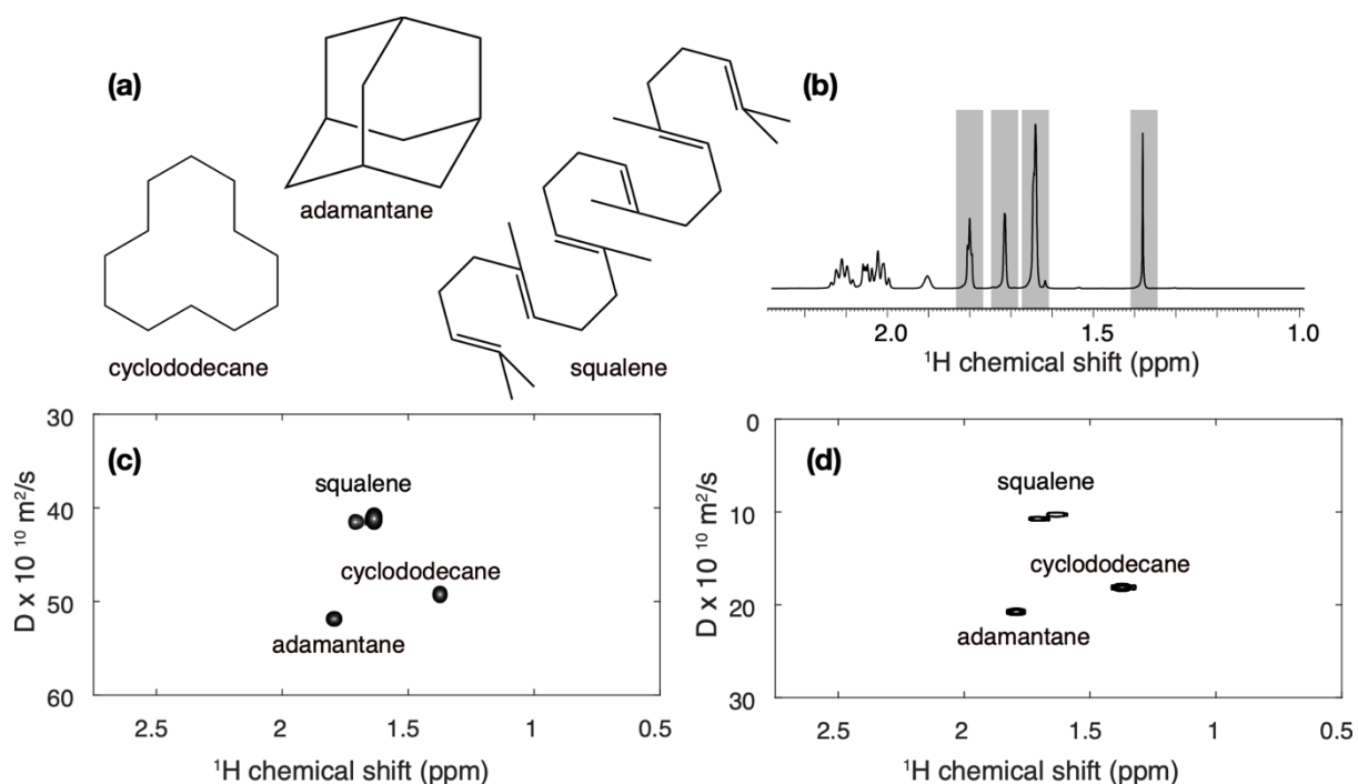
Figure 2 : La convection dans un échantillon peut fausser les mesures de coefficients de diffusion, et son effet doit être compensé. Les trois molécules représentées en (a) sont fréquemment utilisées pour le calibrage en RMN DOSY. L'expérience RMN DOSY ultrarapide initiale donne le résultat (c), dans lequel les coefficients de diffusion sont largement surestimés. L'expérience modifiée pour compenser la convection donne le résultat (d), dans lequel les valeurs mesurées sont correctes. On remarque également que les tâches de corrélations sont plus fines ; l'expérience a une meilleure résolution.
