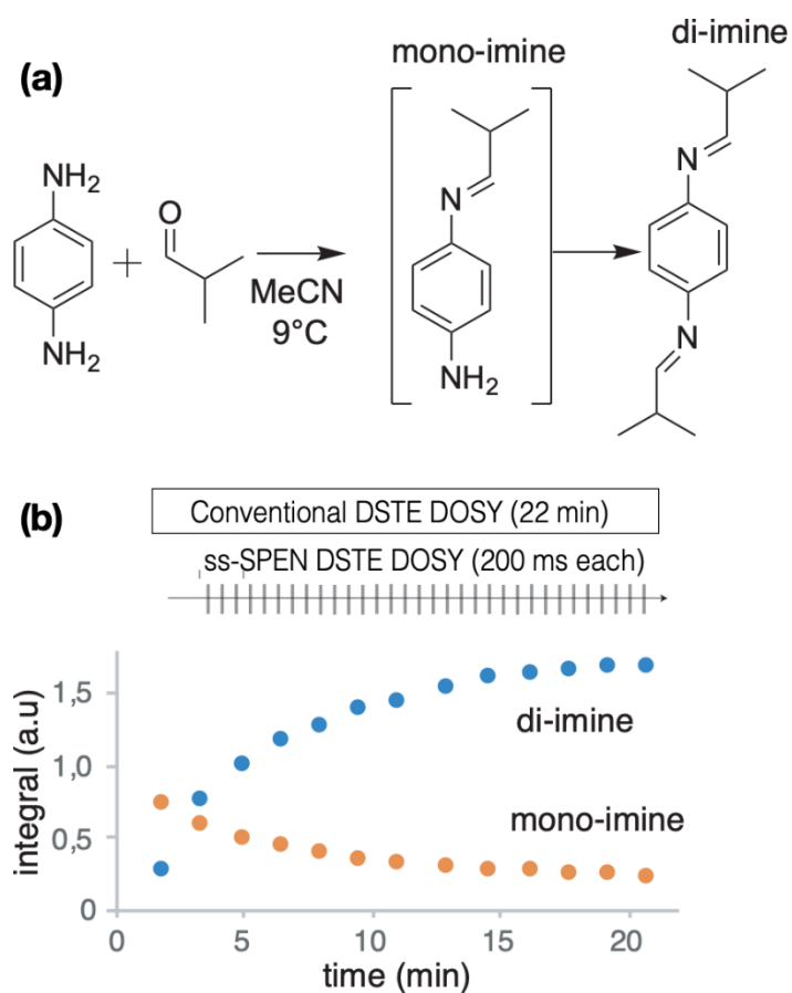
Figure 3 L'expérience RMN DOSY ultrarapide avec compensation de la convection a été utilisée pour suivre la réaction décrite en (a). En (b), on voit l'évolution de la concentration d'un des réactifs, et du produit final, ainsi que la durée de l'expérience DOSY conventionnelle (22 min), et celle de chaque expérience DOSY ultrarapide. Les coefficients de diffusion mesurés sont reportés dans le tableau 1.
