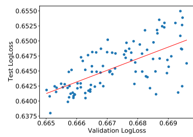
(d) Slope: 1.93 - R^2 : 0.44 - Test year 2019
