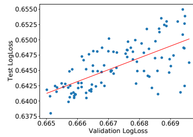
(d) Slope: 1.93 - R^2 : 0.44 - Test year 2019
