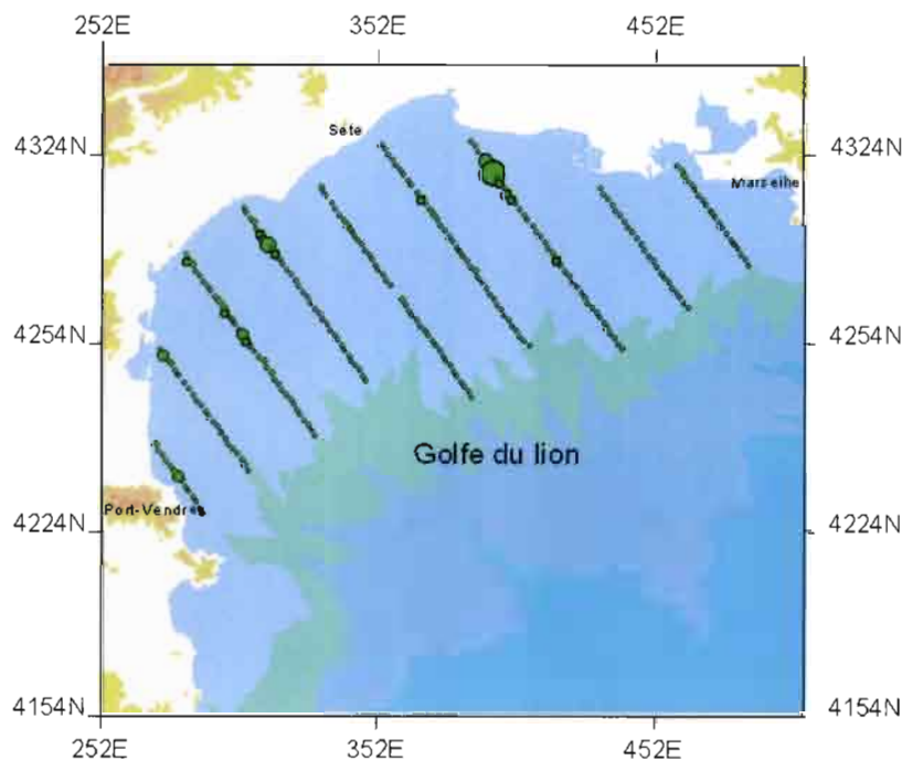
Figure 3 : répartition des énergies calculées au cours de PELMED01, la dimension des cercles est proportionnelle à la densité acoustique calculée.
