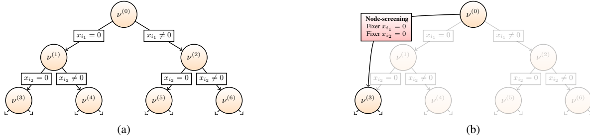
FIGURE 1 – Premiers nœuds explorés dans l’arbre de BnB. Le nœud \nu^{(0)} correspond au problème (P) et chacun de ses descendants correspond au problème (P^\nu) avec différentes variables fixées. (a) Implémentation standard d’un BnB où tous les nœuds sont traités. (b) Impact de l’application des tests de node-screening sur l’arbre de recherche : au nœud \nu^{(0)} , le test (6b) est passé pour les entrées i_1 et i_2 ; on peut donc aller directement au descendant incluant les contraintes “ x_{i_1} = 0 ” et “ x_{i_2} = 0 ”, à savoir \nu^{(3)} . Les nœuds transparents ne sont donc pas explorés.
