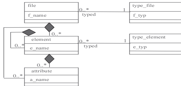
Fig. 6. The meta-model
