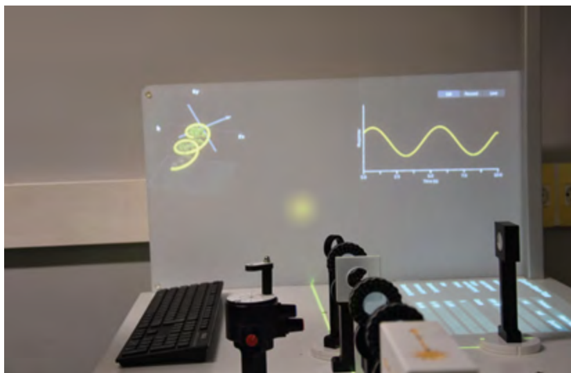
2. Photo montrant certaines représentations lorsque HOBIT est utilisé pour étudier la polarisation de la lumière. Sur l'écran vertical, on observe en haut à gauche l'état de polarisation qui peut être vu en deux dimensions, ou comme ici en trois dimensions. La courbe en haut à droite représente les variations d'intensité que l'on obtient en faisant tourner un polariseur pour analyser l'état de polarisation montré à gauche. Sur le plan horizontal, on devine une zone graphique dans laquelle il est possible de modifier les paramètres du composant sélectionné sur le montage.
